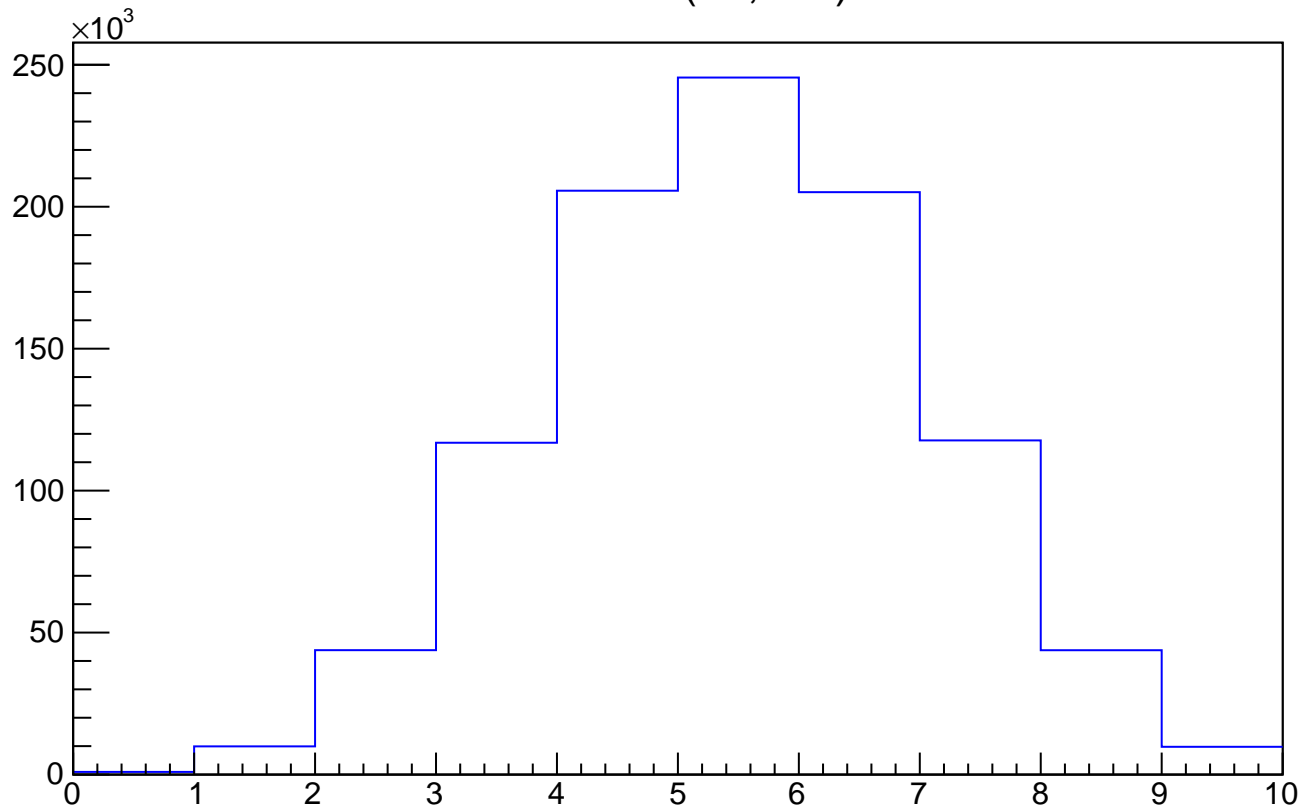
Binomial(10, 0.5)
